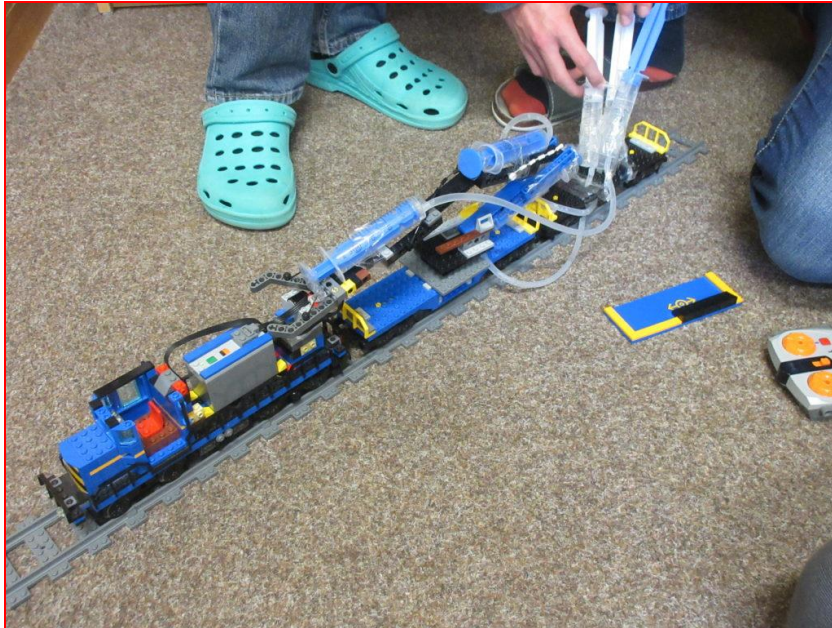
Fyzika - hydrostatické zařízení
